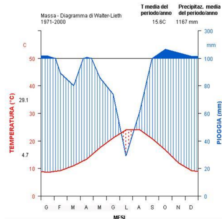
Figura 2 – Diagramma di Walther Lieth
